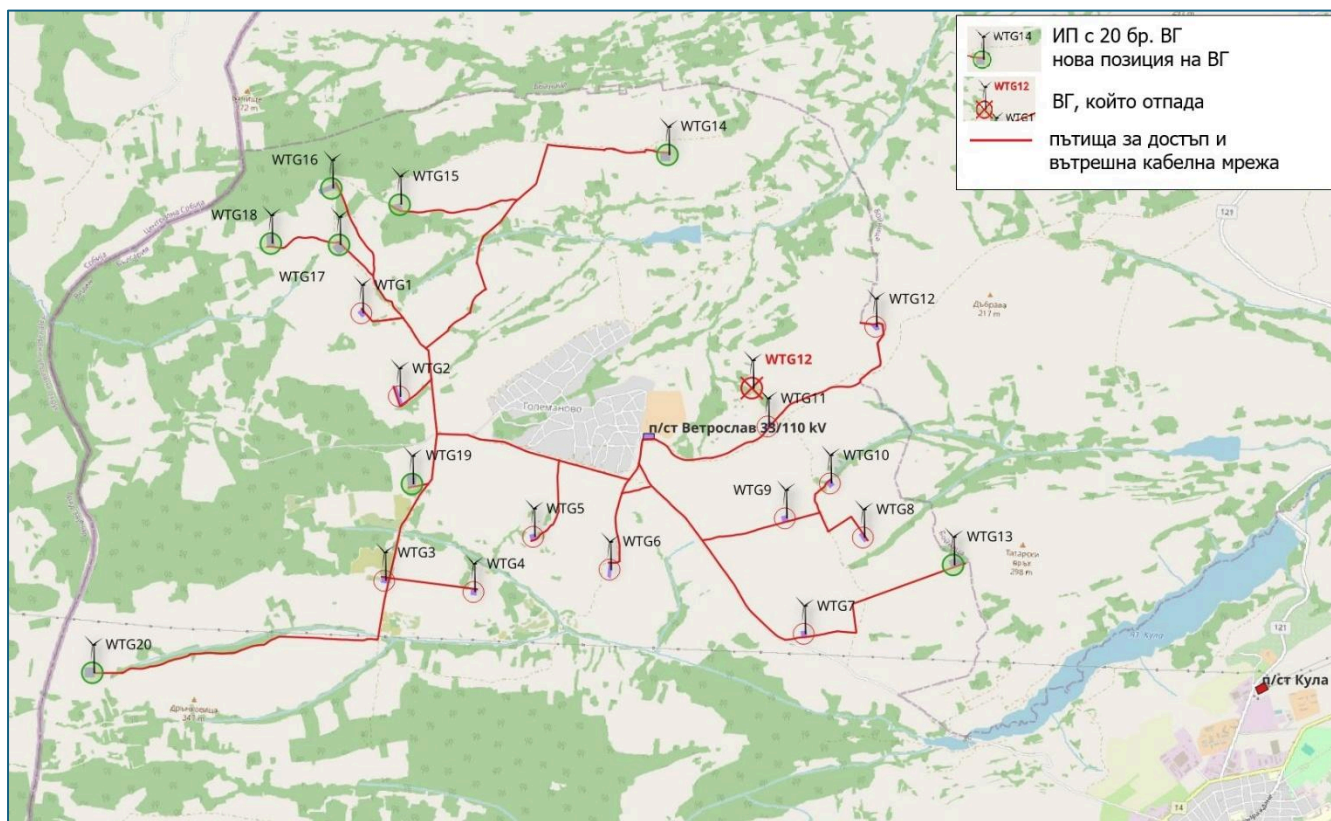
Фигура 6 Пътища за достъп до съоръженията
