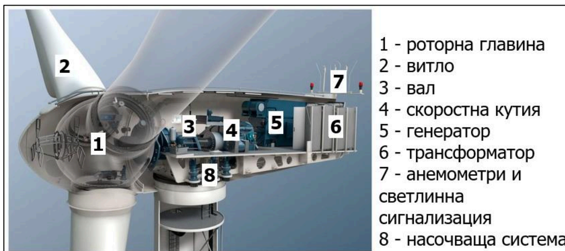
Фигура 2 Разрез на вятърна турбина
