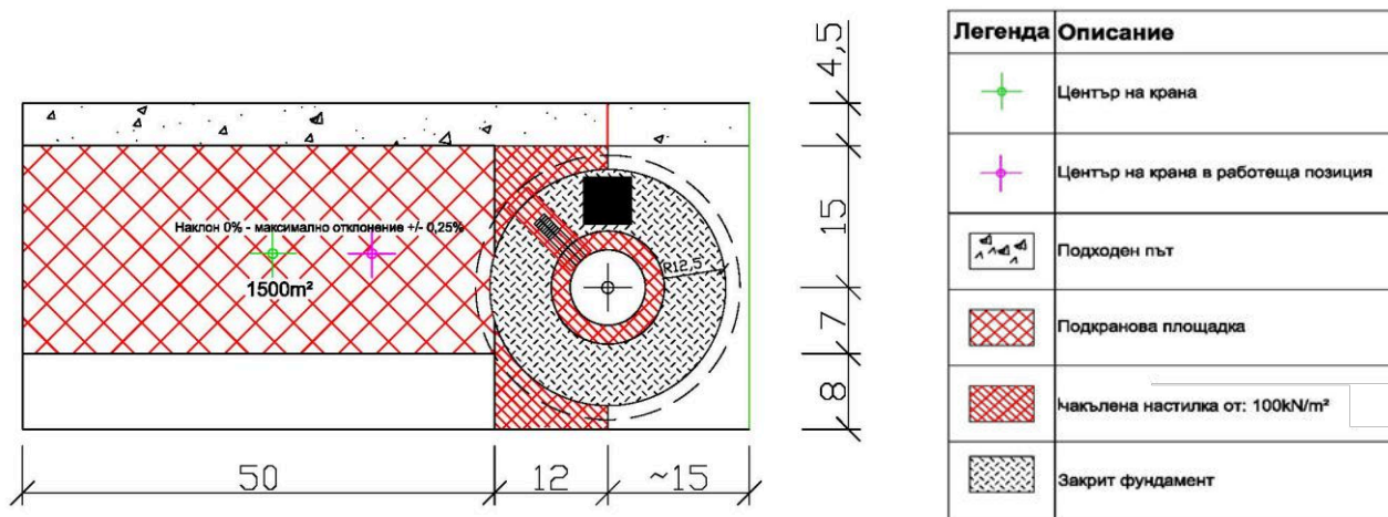
Фигура 4 Примерна схема на фундамент и временна кранова площадка
